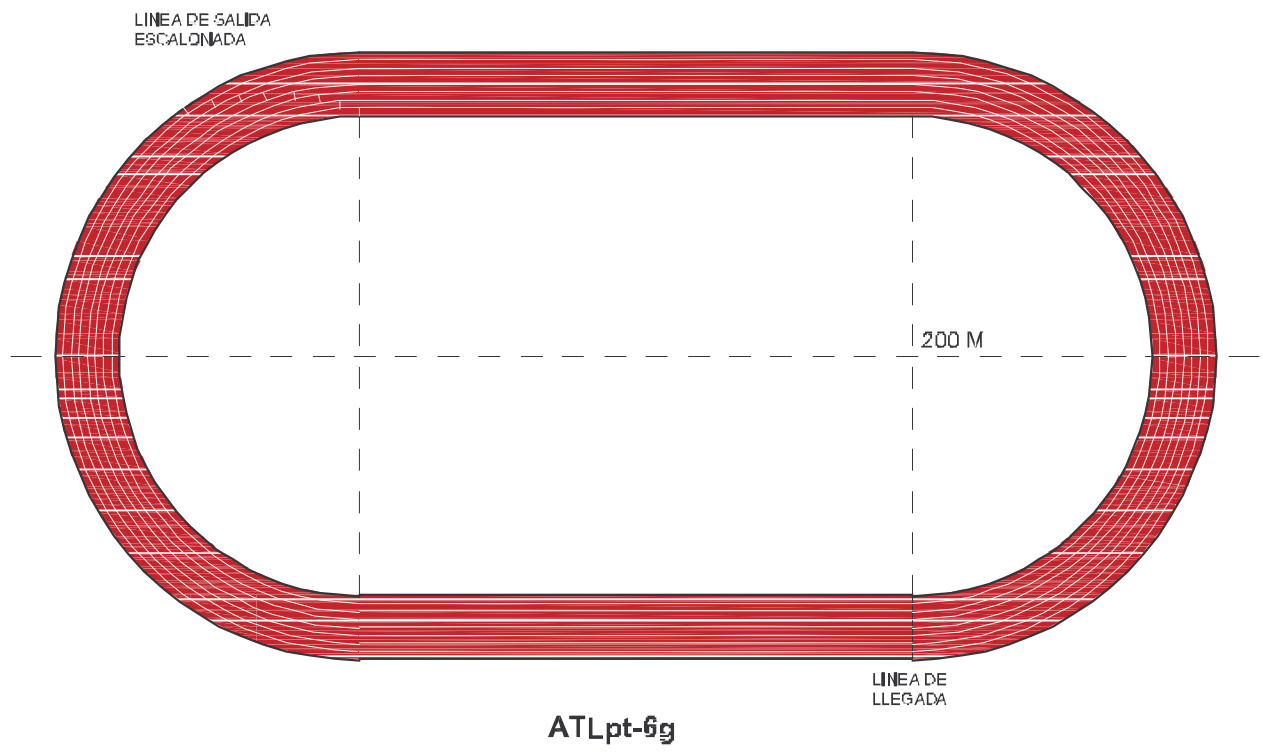
TRAZOS DE COLOCACION DE VALLA
