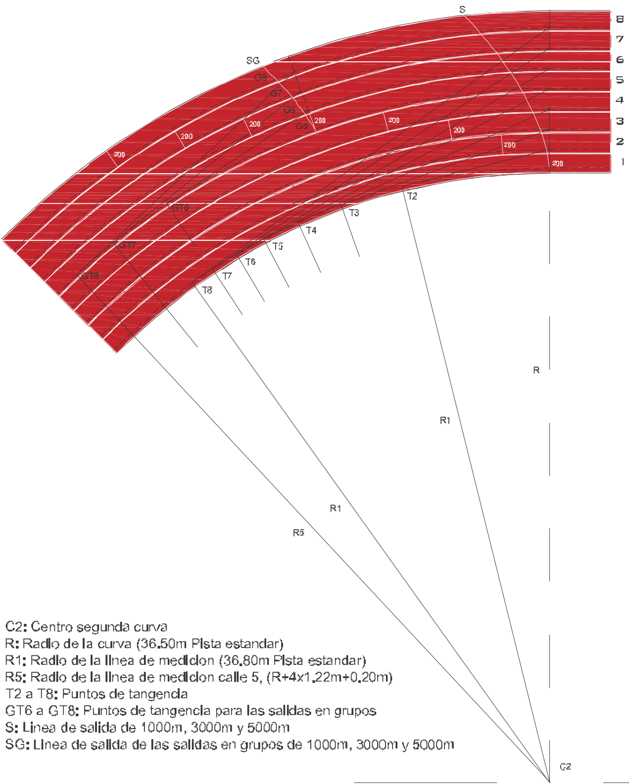
LINEA DE SALIDA EN CURVA Y GRUPOS 1000m, 3000m y 5000m LINEAS DE SALIDA ESCALONADA 200m ATLpt-4b
